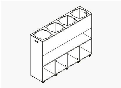
4 Box Planter 1350 open storage W: 1800 x D: 450 x H: 1350 mm (W: 53 x D: 18 x H: 53in)
