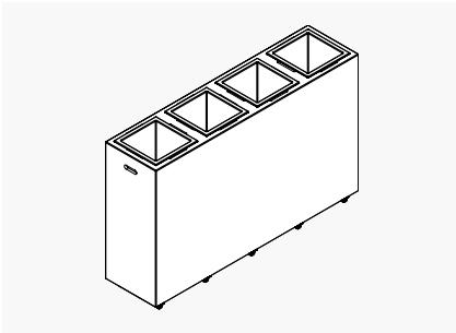
3 Box Planter 1125 W: 1800 x D: 450 x H: 1125 mm (W: 71 x D: 18 x H: 44in)
