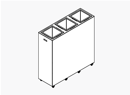
3 Box Planter 1350 W: 1350 x D: 450 x H: 1350 mm (W: 53 x D: 18 x H: 53in)
