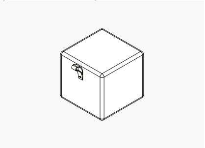
Square 400 W: 400 x D: 400 x H: 410 mm (W: 16 x D: 16 x H: 16in)
