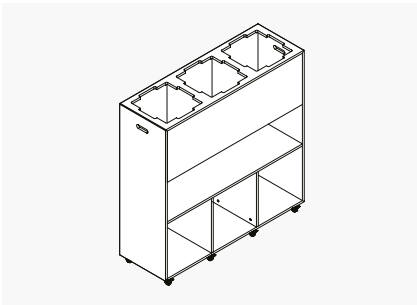
3 Box Planter 1350 open storage W: 1350 x D: 450 x H: 1350 mm (W: 53 x D: 18 x H: 53in)
