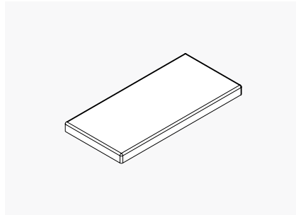
Double Seat Pad W: 850 x D: 400 x H: 50 mm (W: 33 x D: 16 x H: 2in)
