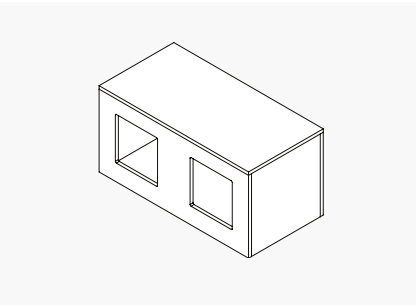
Module 5 Cubby W: 900 x D: 450 x H: 450 mm (W: 35 x D: 18 x H: 18in)
