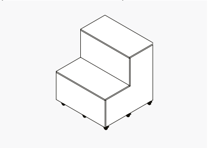
Module 9 with castors W: 900 x D: 900 x H: 940 mm (W: 35 x D: 35 x H: 37in)
