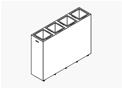
4 Box Planter 1350 W: 1800 x D: 450 x H: 1350 mm (W: 71 x D: 18 x H: 53in)
