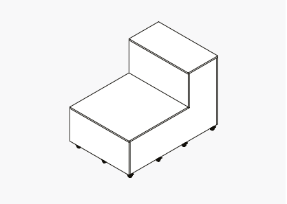
Module 11 with castors W: 900 x D: 1350 x H: 940 mm (W: 35 x D: 53 x H: 37in)
