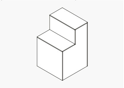
Module 14 W: 900 x D: 900 x H: 1350 mm (W: 35 x D: 35 x H: 53in)
