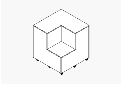
Module 10 with castors W: 900 x D: 900 x H: 940 mm (W: 35 x D: 35 x H: 37in)
