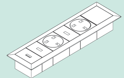
POWER MODULE
